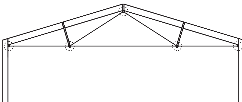
ワーレントラス
