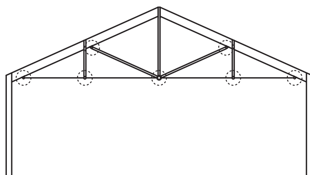
キングポストトラス
